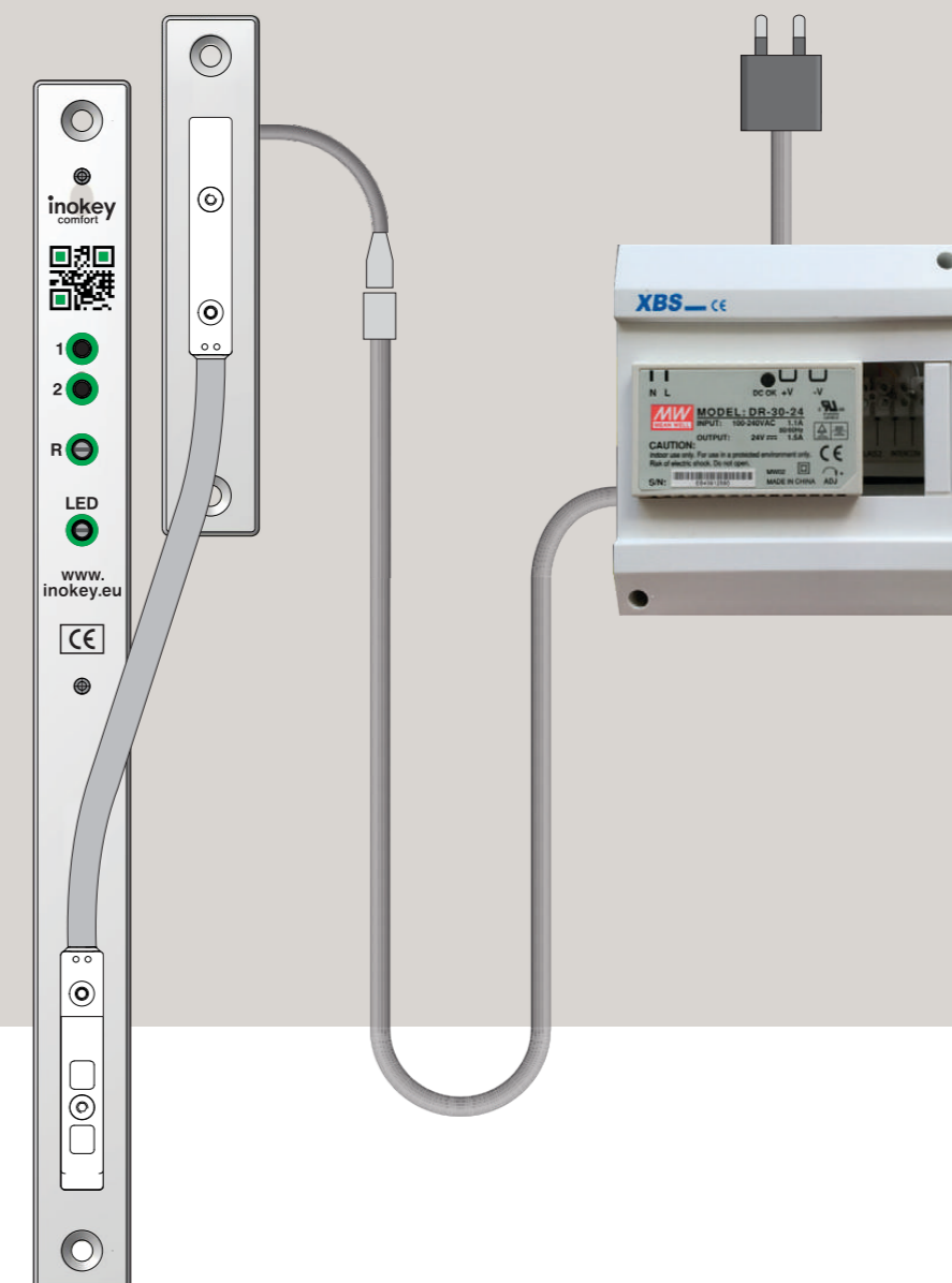
NEU - Kabelübergang und Steuereinheit
